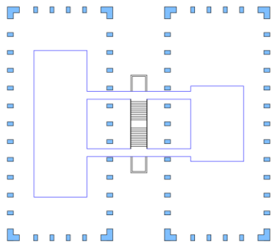
Planta baja y 2° piso
