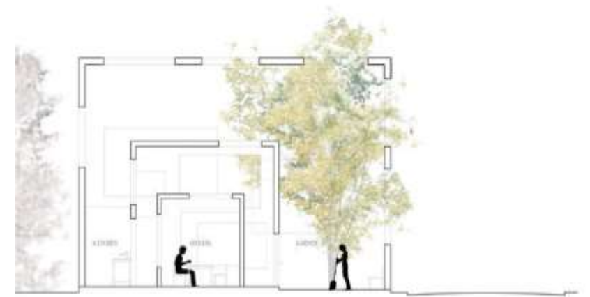
Casa N Sou Fujimoto
