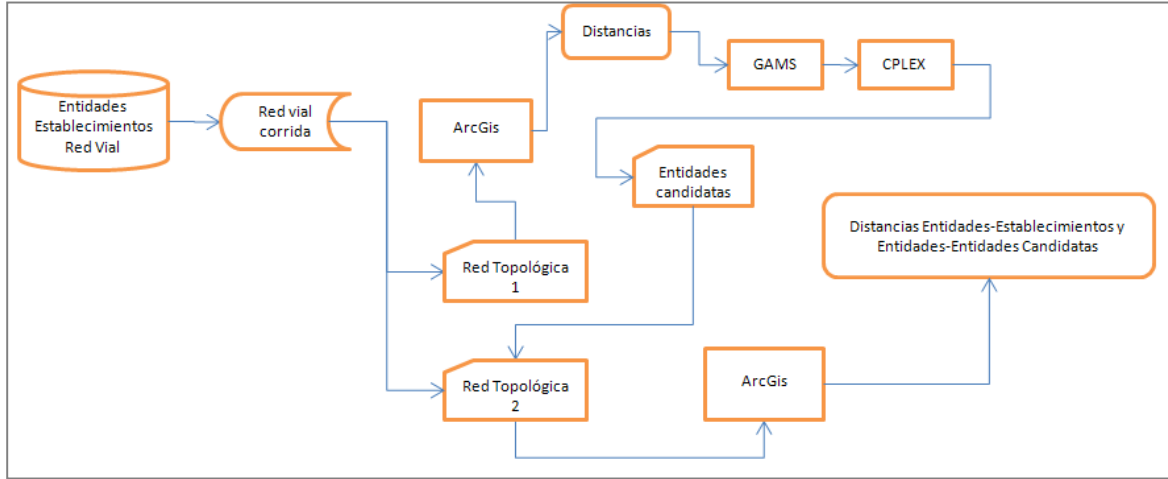
Figura 3. Sub-modelo 1. Calculo de distancias entre entidades y establecimientos y entidades candidatas
