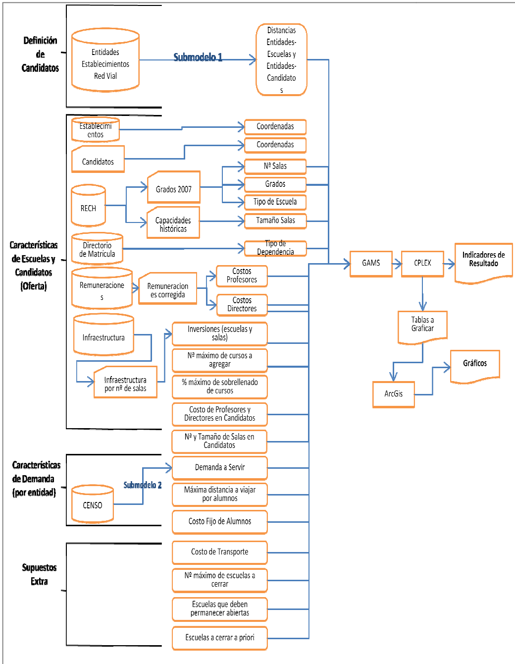
Figura 2. Esquema de los procesos para la aplicación el modelo de localización.
