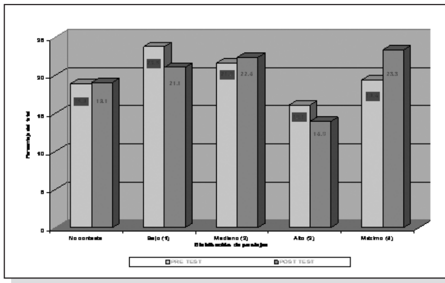
Gráfico 12: Distribución de los resultados Test Curricular Ítem 3
