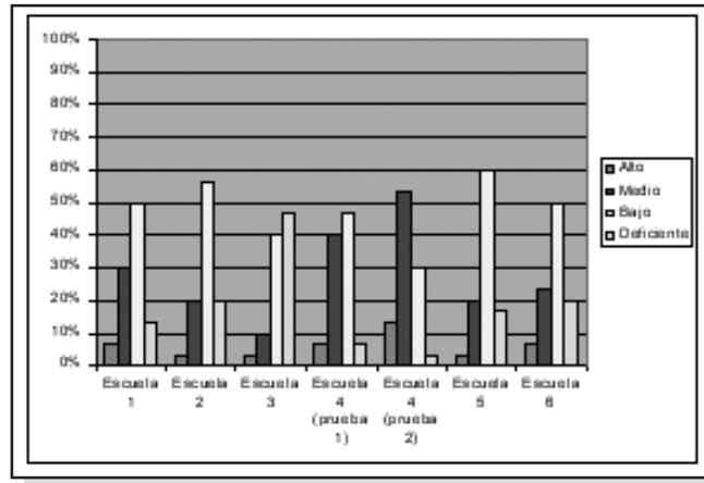
Gráfico.- Resultados de las evaluaciones aplicadas por el profesor
