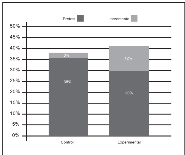
Gráfico 4-1 Resultados del Pre-test e incrementos obtenidos en grupo experimental y control
