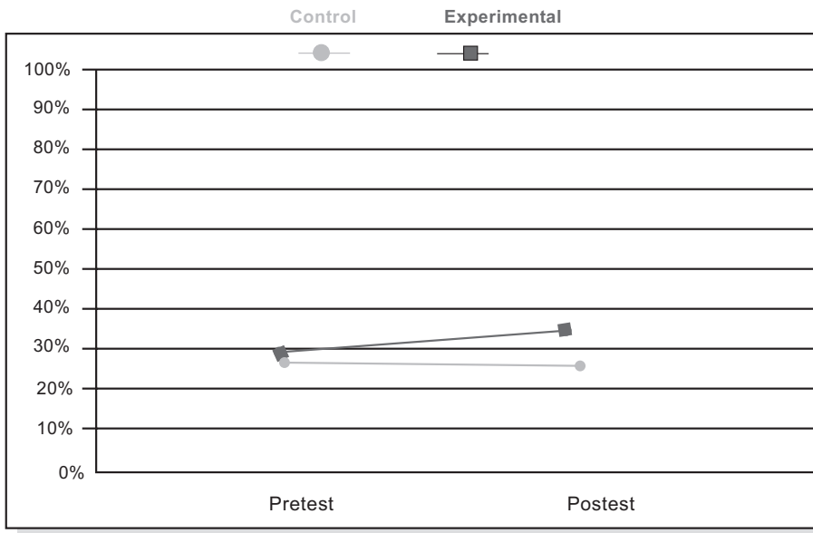
Gráfico1. Resultados del pre-test y pos-test obtenidos en el grupo experimental y control.
