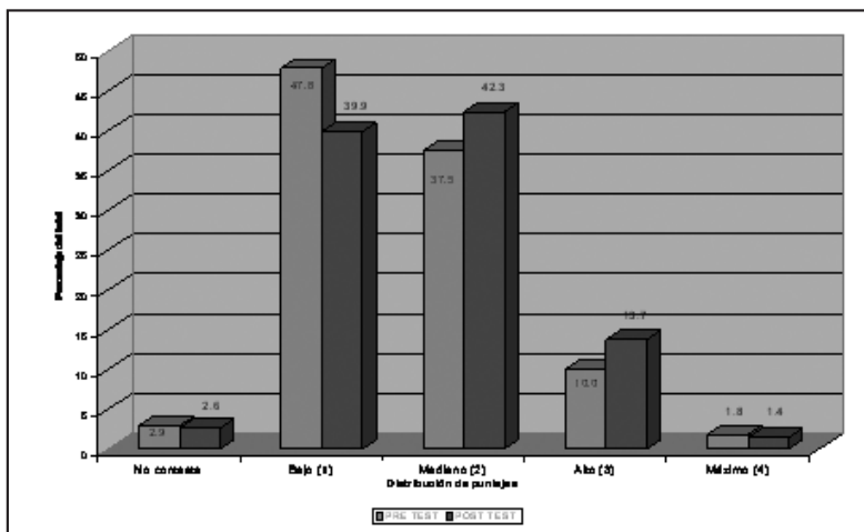
Gráfico 9: Distribución de los resultados Test Curricular Ítem 1 Actividad 2
