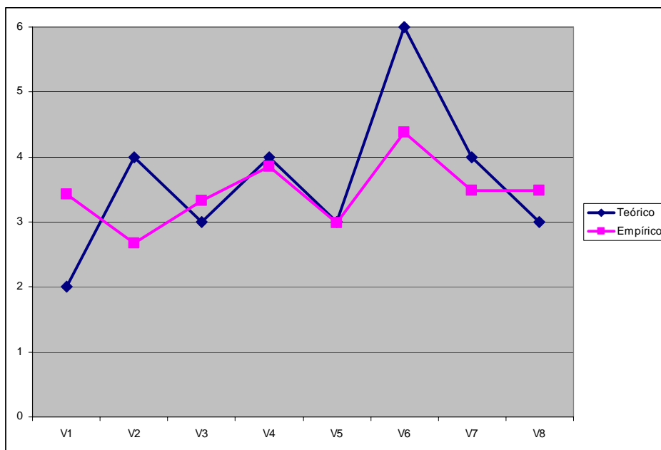
Gráfico N° 18 Comparación Vectores Teóricos y Observados en Contabilidad
